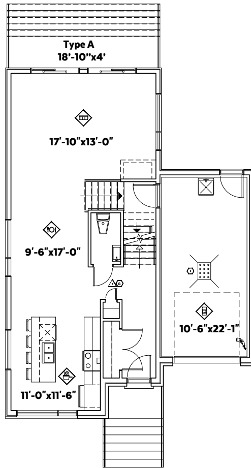
PLAN DU REZ-DE-CHAUSSEE
