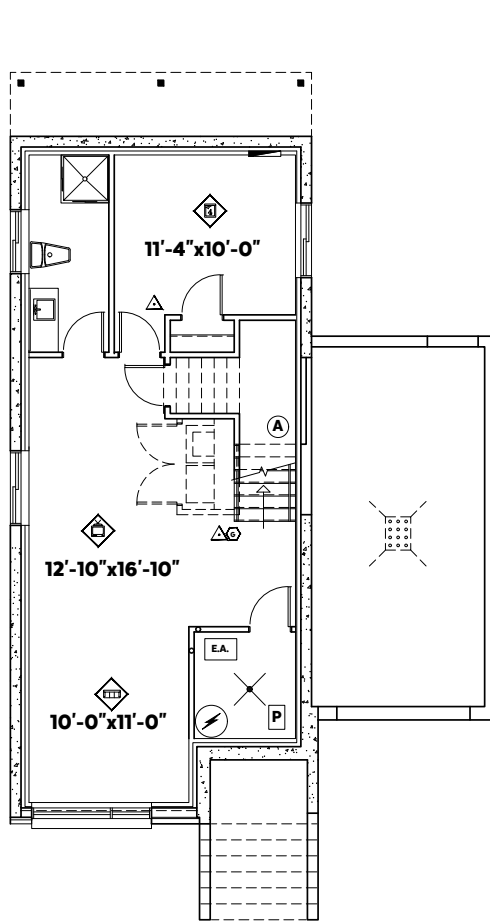
PLAN DU SOUS-SOL
